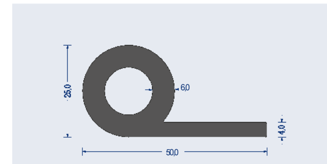
Artikel-Nr. 1540.5252 EPDM · 60° ShoreA · schwarz VE: Bund á 25m
