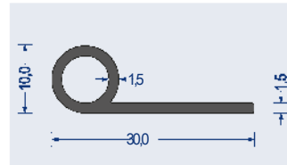
Artikel-Nr. 1540.5104 EPDM · 60° ShoreA · schwarz VE: Bund á 50m
