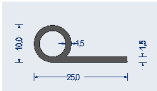
Artikel-Nr. 1540.5101 EPDM · 65° ShoreA · schwarz VE: Bund á 50m
