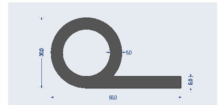
Artikel-Nr. 1540.5301 EPDM · 65° ShoreA · schwarz VE: Bund á 25m
