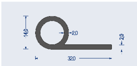
Artikel-Nr. 1540.5141 EPDM · 65° ShoreA · schwarz VE: Bund á 50m
