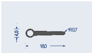
Artikel-Nr. 1540.5049 EPDM · 50° ShoreA · schwarz VE: Bund á 100m
