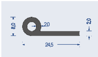
Artikel-Nr. 1540.5084 EPDM · 70° ShoreA · schwarz VE: Bund á 50m
