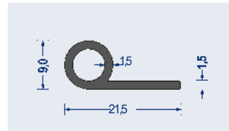
Artikel-Nr. 1540.5094 EPDM · 70° ShoreA · schwarz VE: Bund á 50m
