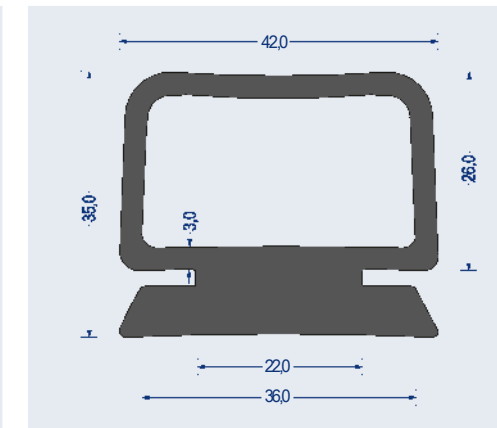
Artikel-Nr. 1540.3049 EPDM · 60° ShoreA · schwarz VE: Länge á 8m 543.3019 / 540.3079 / 540.3049 Aluminium blank VE: Länge á 5m Mindestmenge 10m
