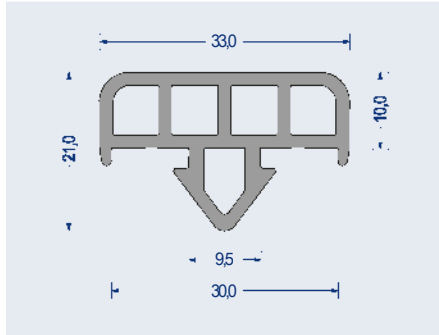
Artikel-Nr. 1547.4256 PVC · 70° ShoreA · grau VE: Bund á 30m
