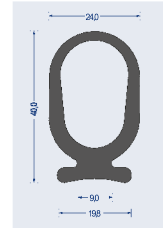
Artikel-Nr. 1540.3139 EPDM · 70° ShoreA · schwarz VE: Bund á 25m
