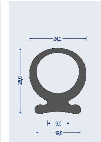
Artikel-Nr. 1540.3129 EPDM · 70° ShoreA · schwarz VE: Bund á 25m
