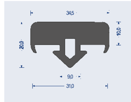
Artikel-Nr. 1540.4239 EPDM · 70° ShoreA · schwarz VE: Bund á 25m
