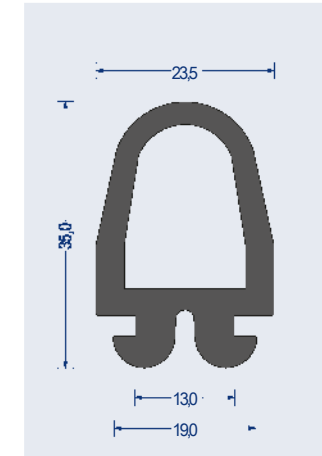
Artikel-Nr. 1540.3069 EPDM · 65° ShoreA · schwarz VE: Bund á 25m
