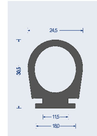
Artikel-Nr. 1540.3079 EPDM · 65° ShoreA · schwarz VE: Bund á 50m
