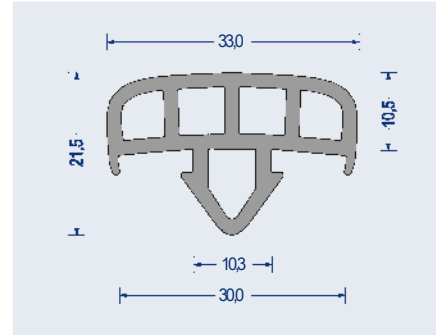
Artikel-Nr. 1547.4356 PVC · 85° ShoreA · grau VE: Bund á 30m
