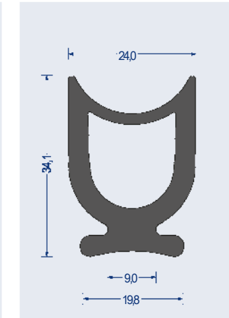
Artikel-Nr. 1540.3169 EPDM · 70° ShoreA · schwarz VE: Bund á 25m
