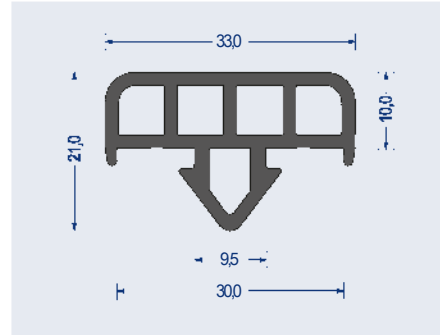
Artikel-Nr. 1547.4259 PVC · 70° ShoreA · schwarz VE: Bund á 30m
