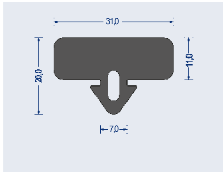
Artikel-Nr. 1540.4109 EPDM · 65° ShoreA · schwarz VE: Bund á 25m
