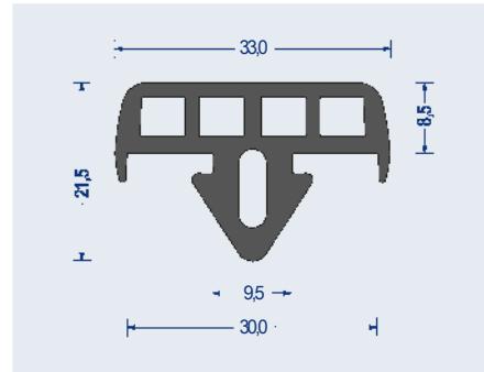
Artikel-Nr. 1540.4409 EPDM · 70° ShoreA · schwarz VE: Bund á 25m
