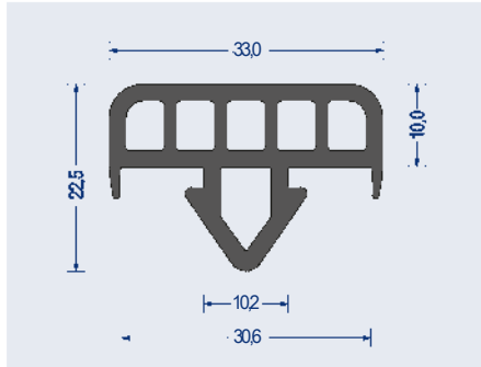
Artikel-Nr. 1540.4510 EPDM · 60° ShoreA · schwarz VE: Bund á 25m
