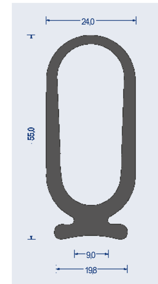
Artikel-Nr. 1540.3149 EPDM · 70° ShoreA · schwarz VE: Bund á 15m
